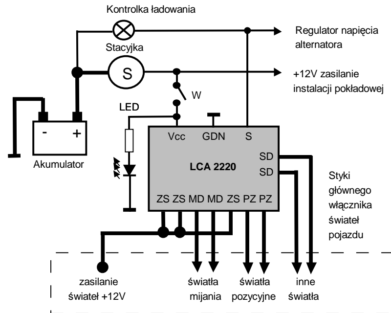
Rys. Schemat podłączenia LCA 2220 do instalacji samochodu
