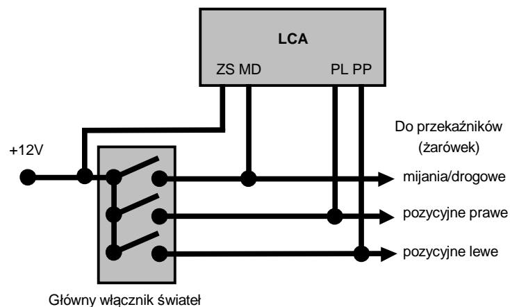
Rys. Ogólna zasada podłączenia LCA do instalacji oświetleniowej pojazdu
