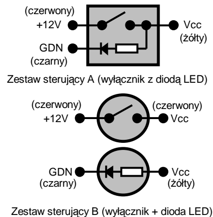
Rys. Schemat wewnętrzny LCA 2220 i wyprowadzenia zestawu sterującego
