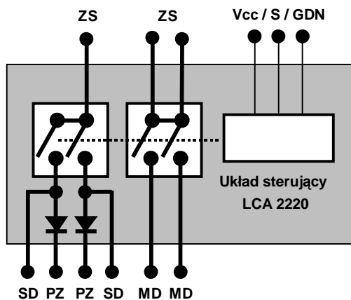
Rys. Schemat wewnętrzny LCA 2220 i wyprowadzenia zestawu sterującego
